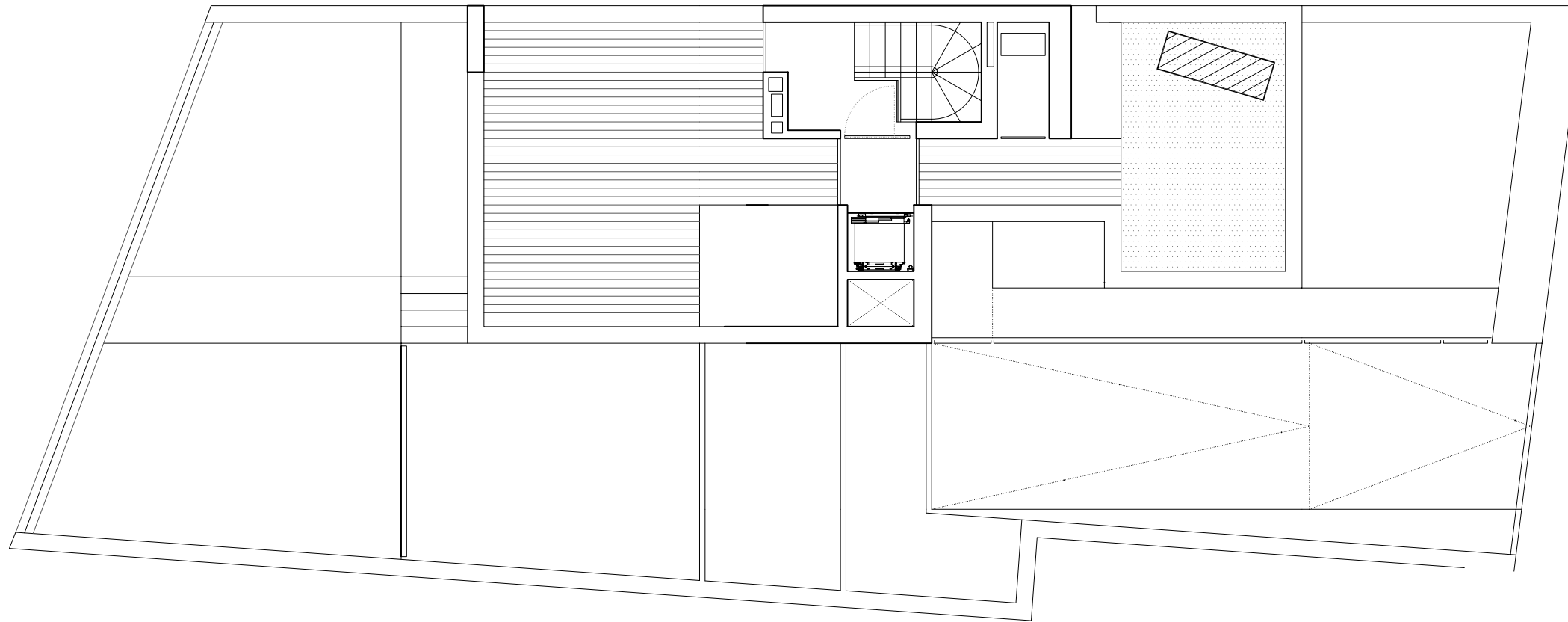
PLANTA DE CUBIERTA SECCIONADA
